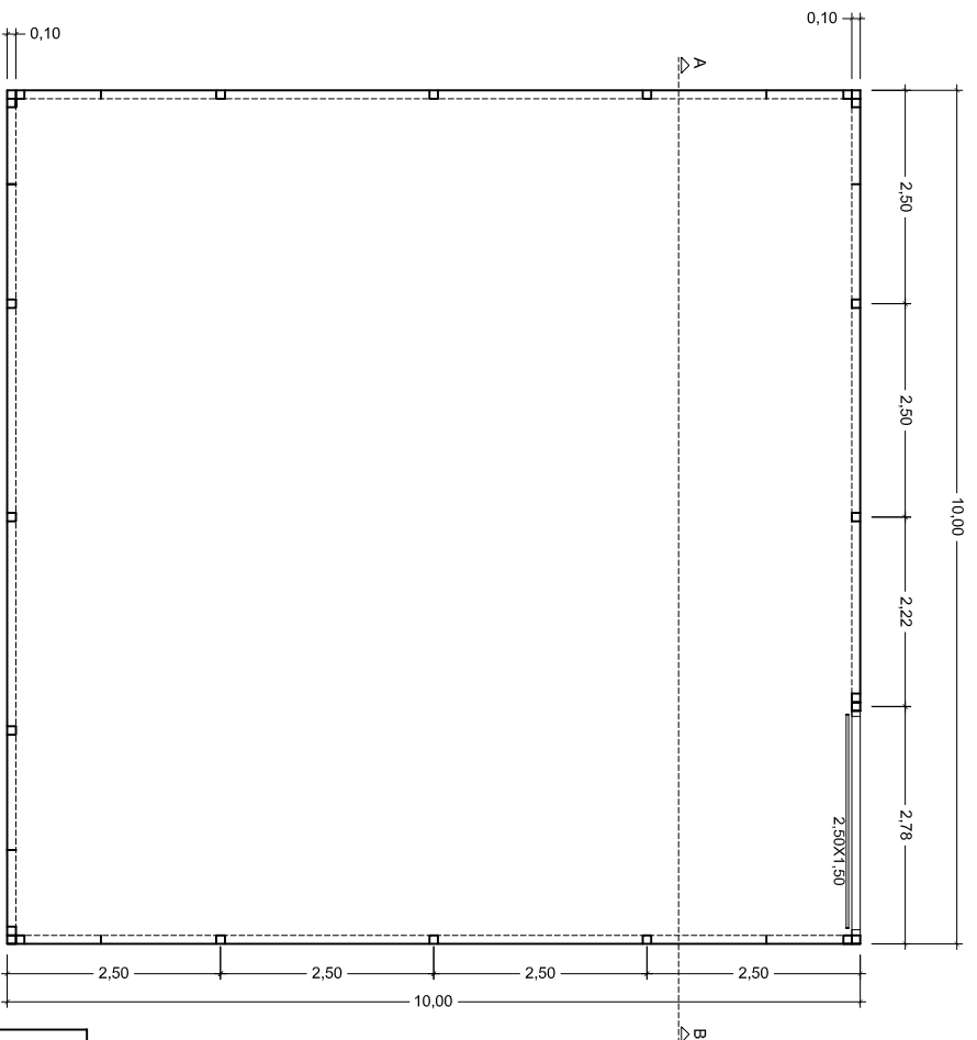
PLANTA BAIXA
