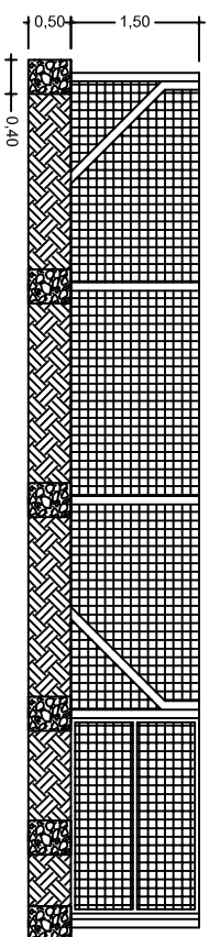
CORTE AB Esc.: 1/75
