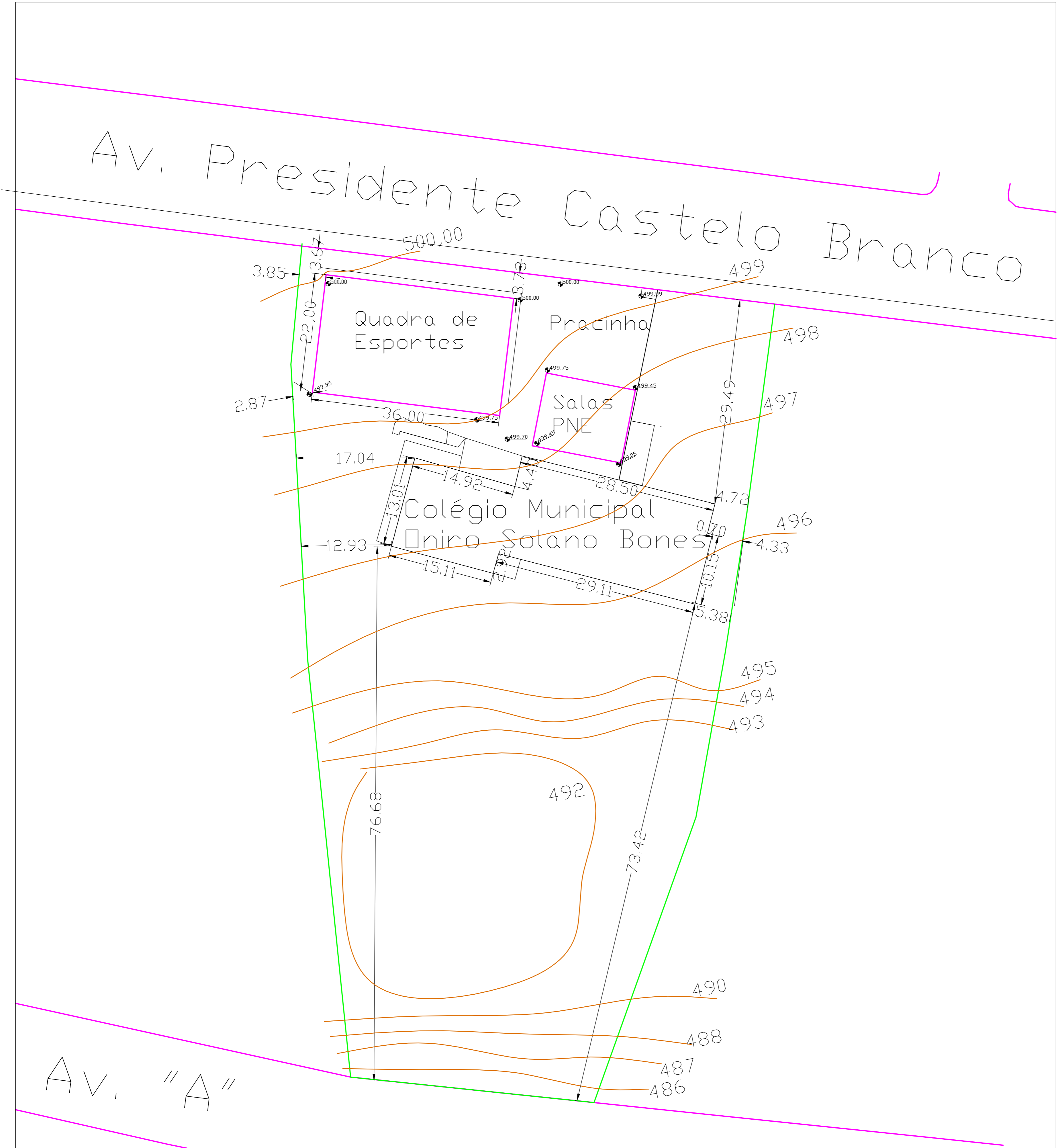
Croqui Planta de Locação Curvas de nível
